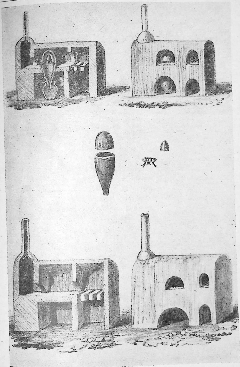
FIG. 665.—HORNOS DE REDUCCIÓN DE ORO Y PLATA USADOS EN CHILE (1826). (Litografía de Baynes, según croquis de John Miers.)
