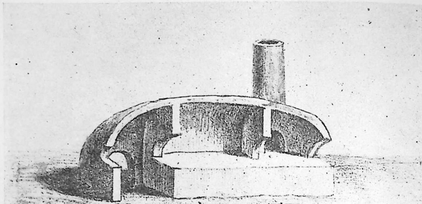
FIG. 663.—PROCEDIMIENTOS METALÚRGICOS EMPLEADOS EN CHILE: HORNO DE FUNDICIÓN DE COBRE, SEGÚN MIERS (1826).
